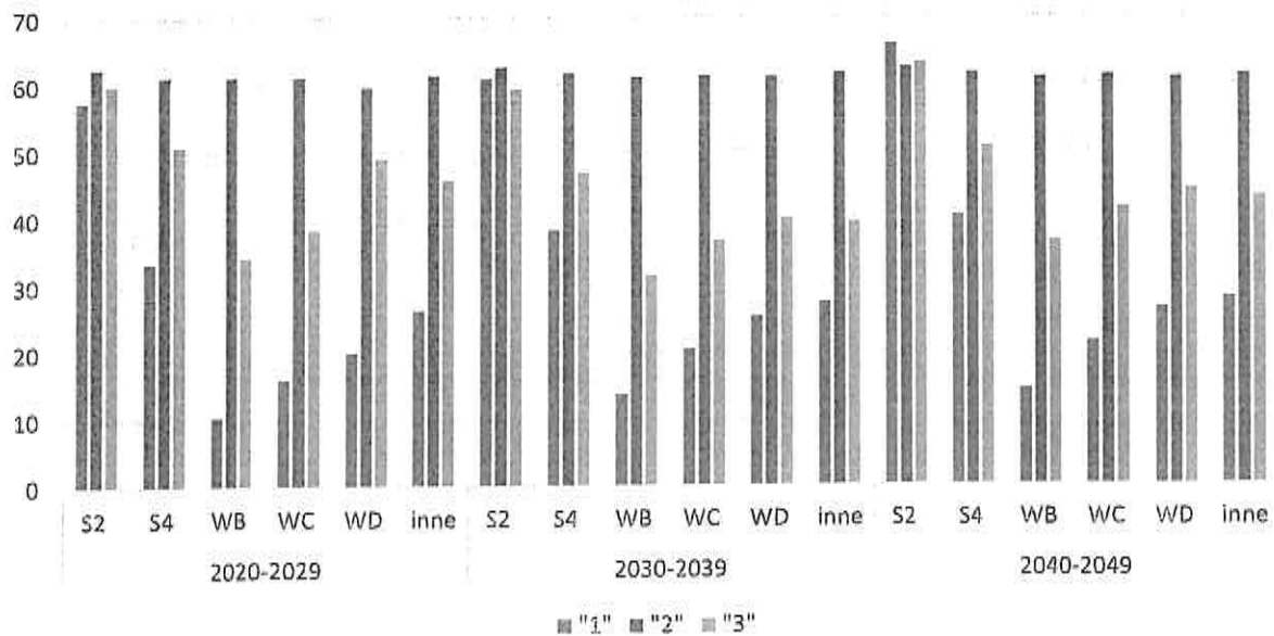
Rysunek 8 Zmniejszenie udziału poszczególnych grup sortymentów scenariusza „1”, „2”, „3” w odniesieniu do „0”
