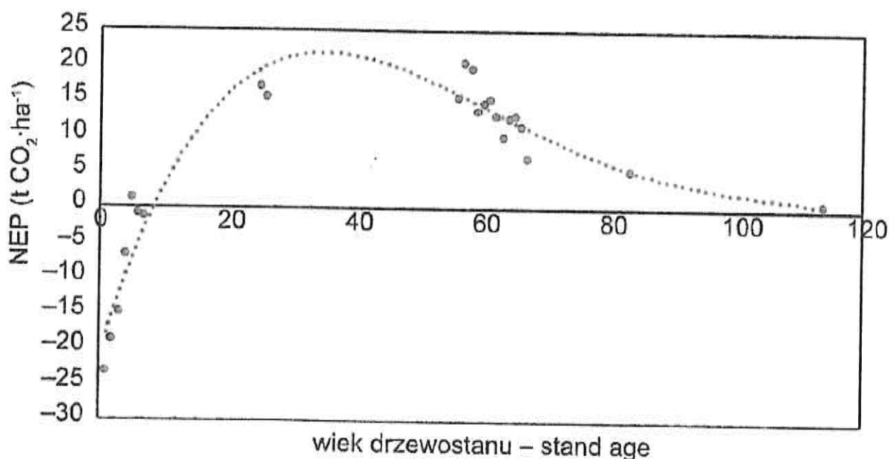
Rysunek 20 Zdolność pochłaniania CO 2 w drzewostanach sosnowych w Polsce w zależności od wieku (Źródło: Olejnik i Małek 2020 s. 395)
